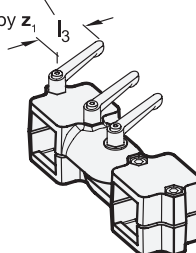
Regulowana dźwignia ręczna GN 911
